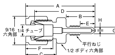
ハネウェル製 DP トランスミッタ用キャリブレーション・アダプター
